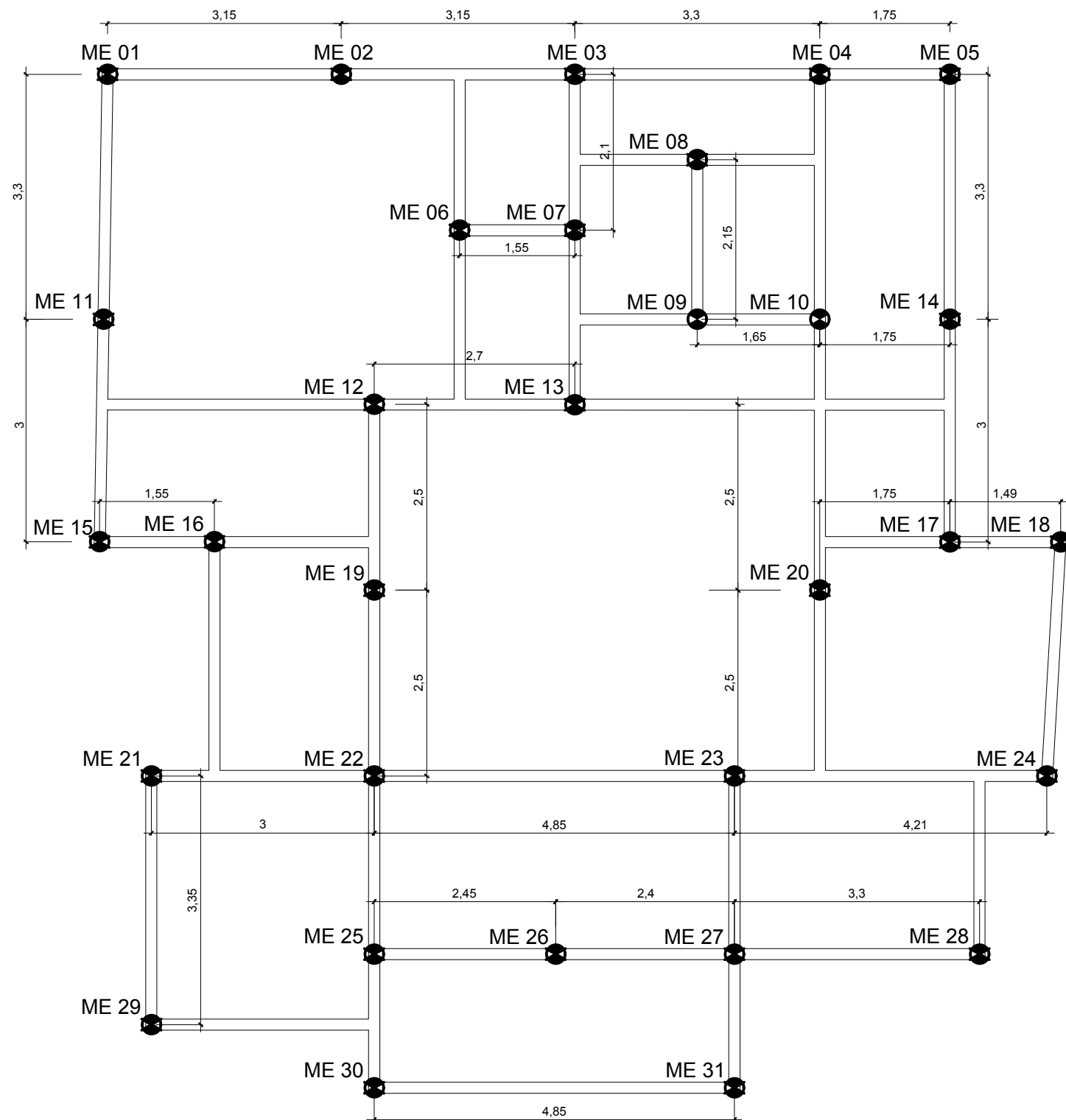
PLANTA BAIXA MICRO-ESTACAS
