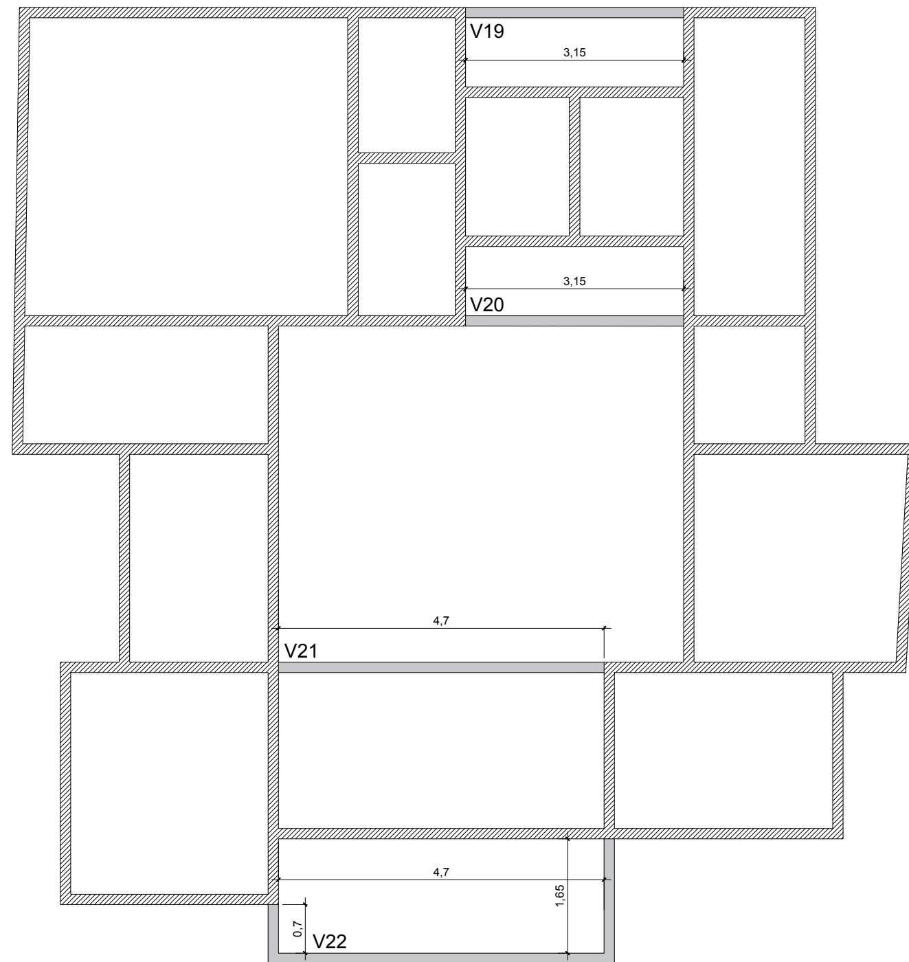
PLANTA BAIXA VIGA RESPALDO
