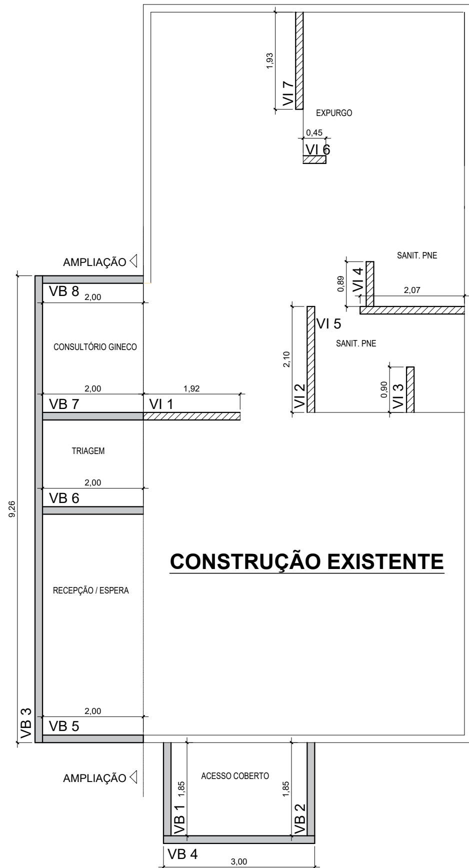
PLANTA BAIXA VIGA BALDRAME UNIDADE BÁSICA DE SAÚDE - DISTRITO DE CAMPO BOM ÁREA : 121,36m 2
