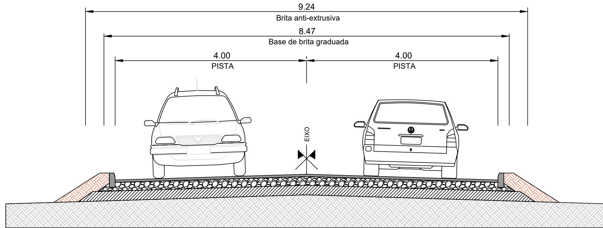
SEÇÃO TIPO DE PAVIMENTAÇÃO SEM ESCALA
